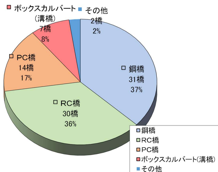
図 3 橋種別の橋梁数（径間数）
