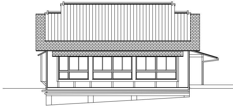
東立面圖 1:100
