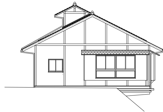
南立面圖 1:100
