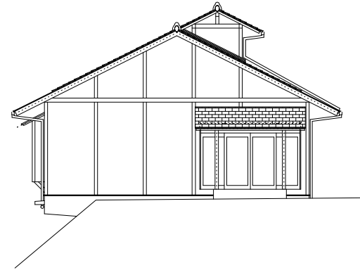
北立面圖 1:100
