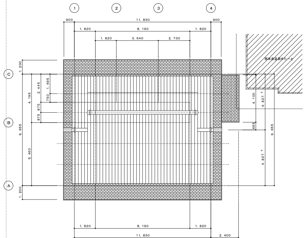
屋根伏図 1:100
