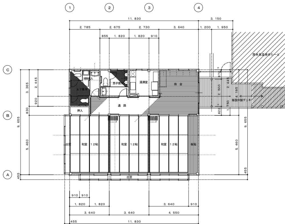
平面図 1:100
